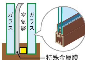
LOW-E ガラスの 断面図
